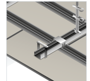
Alternatieve afhangingsmethode met Directafhangers
