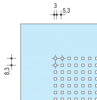
Micro M1 (foratura quadrata) 3x3
