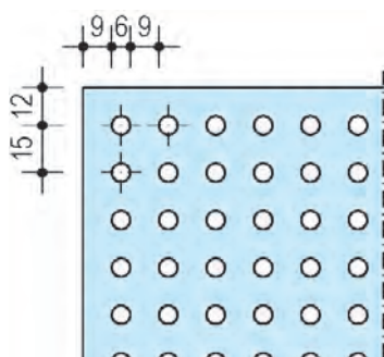
Unity 6 (foratura rotonda) Ø 6
