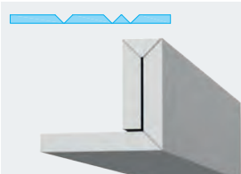
1x 45° + 1x 90° Fresature a V
