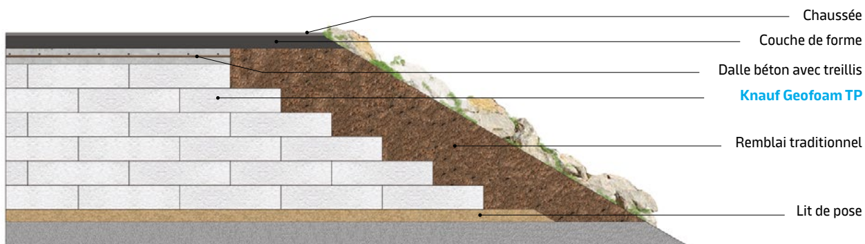
Illustration d'un remblai pour voirie
