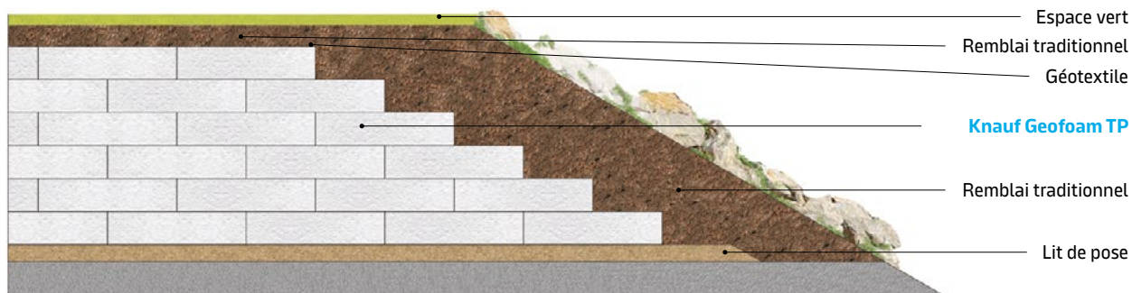
Illustration d'un remblai paysager
