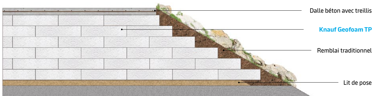
Illustration d'un remblai piétonnier ou terrasse
